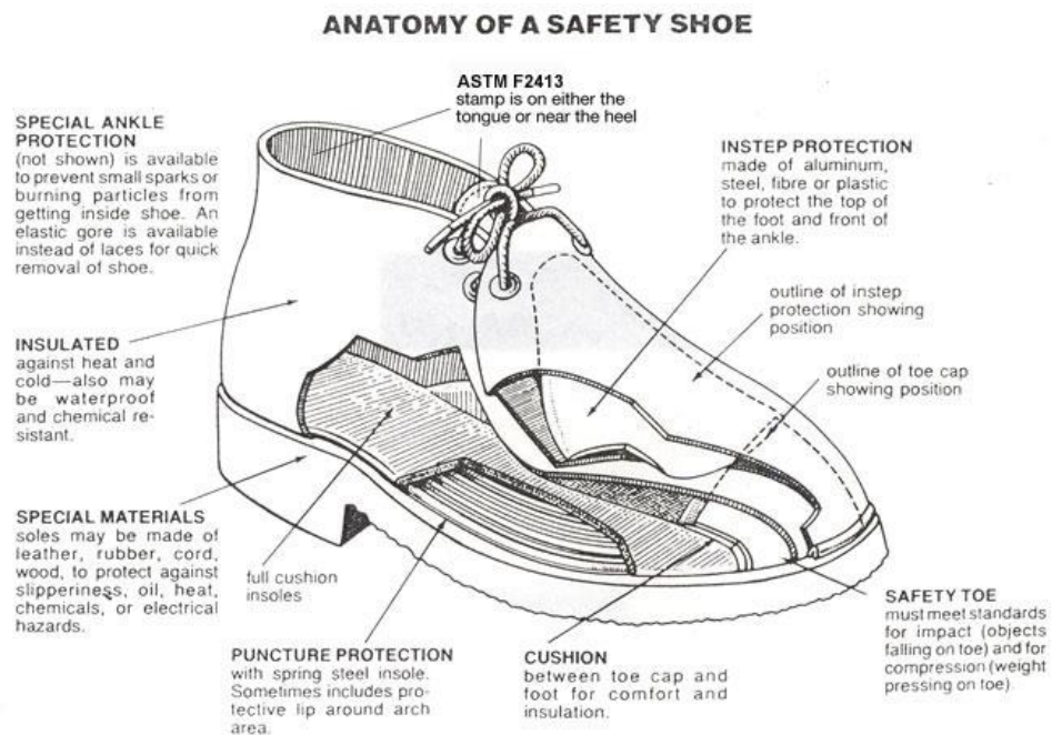
Gambar 9. Sepatu Kerja
