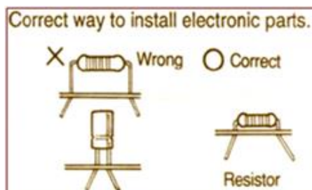
Gambar 41 Pemasangan komponen
