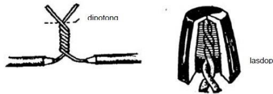
Gambar 18. Sambungan kabel cara ekor babi ( pig tail )
