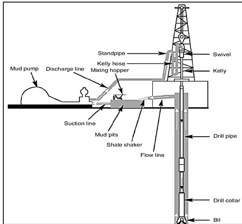
Gambar 4.31. Sistem Sirkulasi
