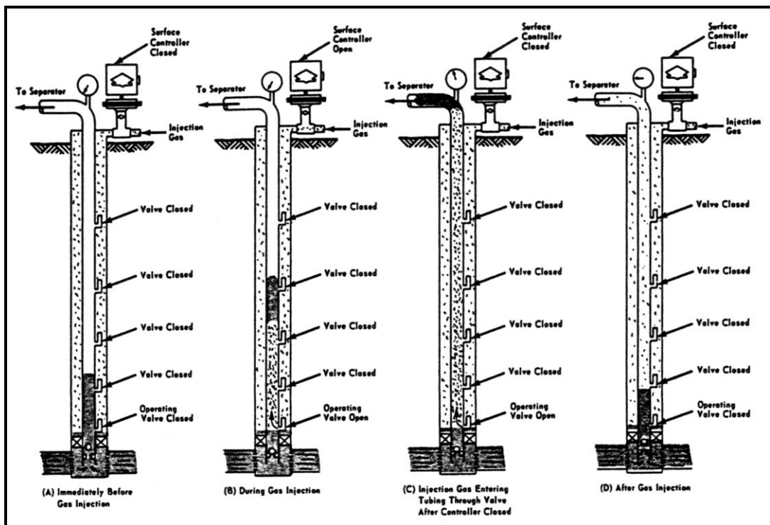
Gambar 8.7. Siklus Operasi Aliran Intermittent untuk Instalasi-Tertutup Konvensional
