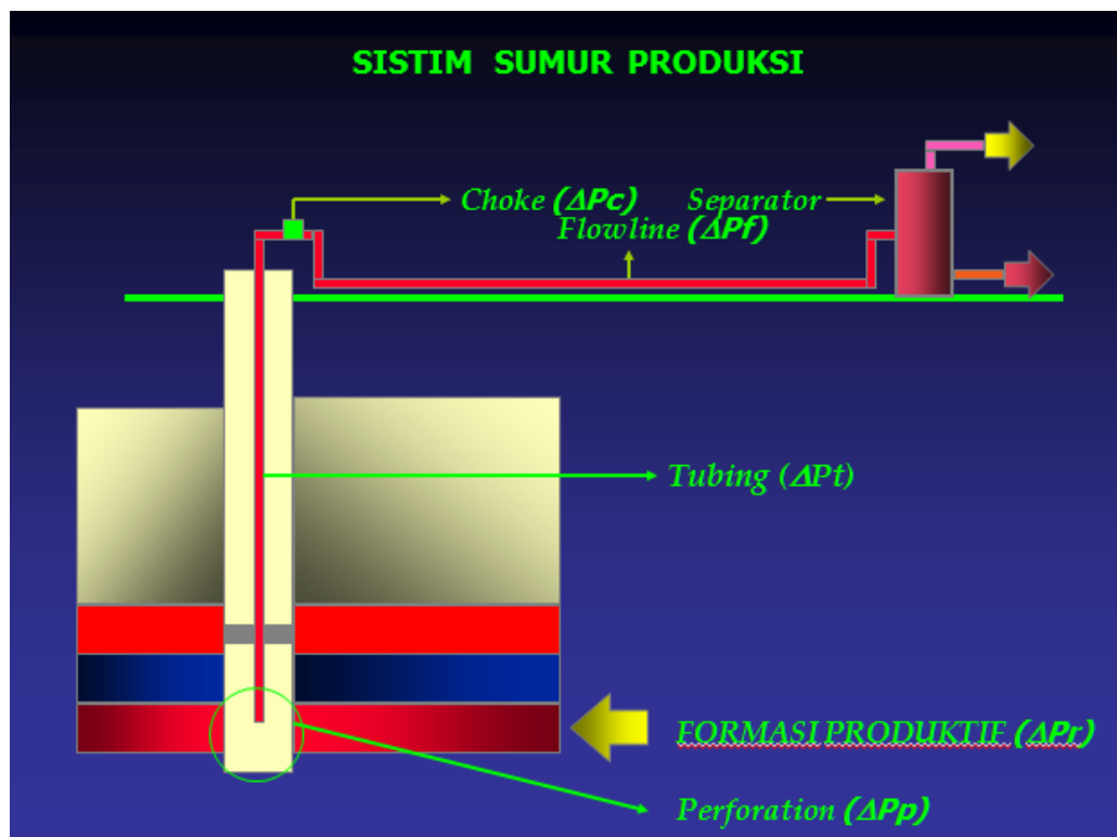
Gambar 8.1. Sistem Sumur Produksi
