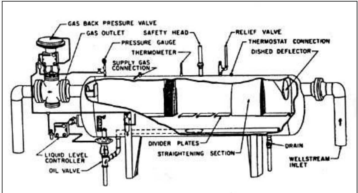
Gambar 8.16. Separator Horizontal Bertabung Tunggal
