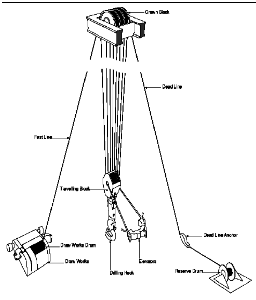
Gambar 4.2. Sistem Angkat ( hoisting system )
