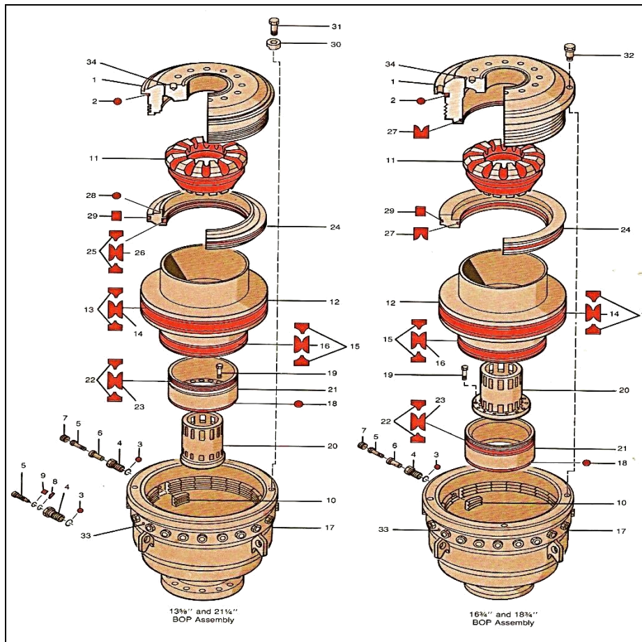
Gambar 4.40. Bagian-Bagian dari Annular Preventer
