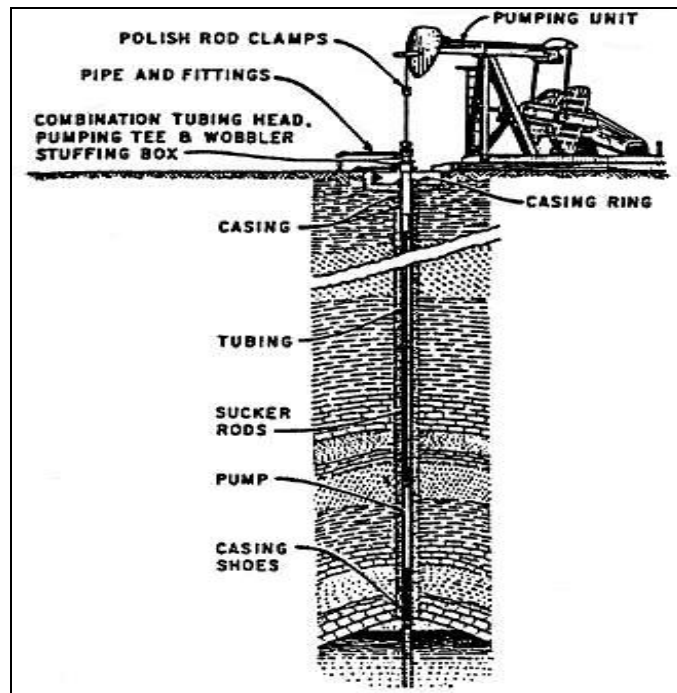
Gambar 8.8. Sistem Pemompaan Beam
