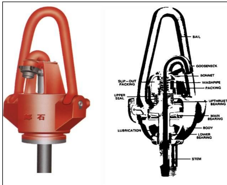
Gambar 4.11. Swivel
