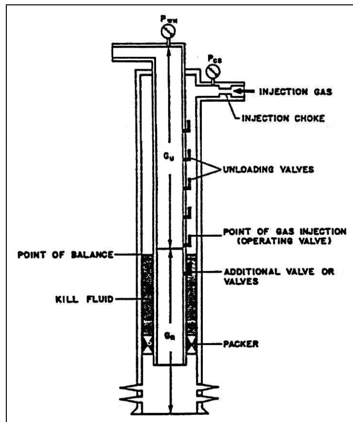
Gambar 8.6. Operasi Gas-Lift Aliran Kontinyu
