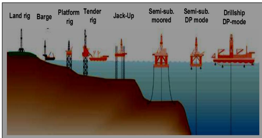
Gambar 3.5. Onshore dan Offshore drilling
