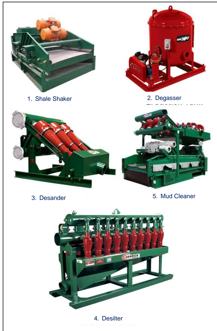
Gambar 4.35. Peralatan Pengkondisi Lumpur Pengeboran
