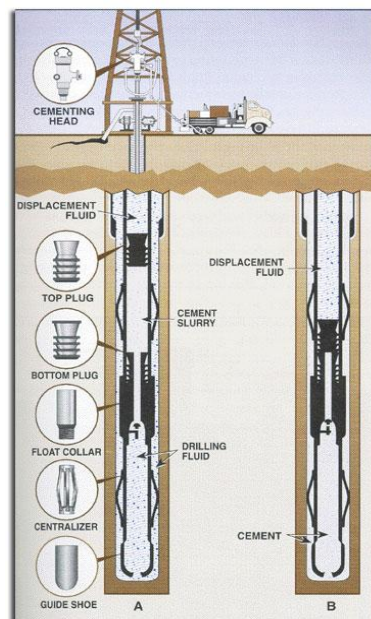
Gambar 5.7. Ilustrasi Operasi Penyemenan
