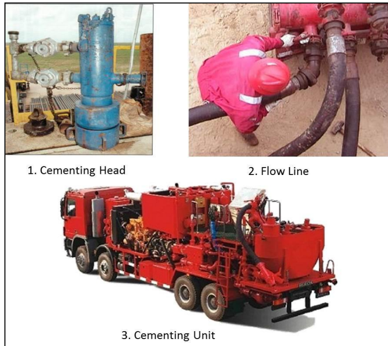
Gambar 5.9. Peralatan di atas permukaan
