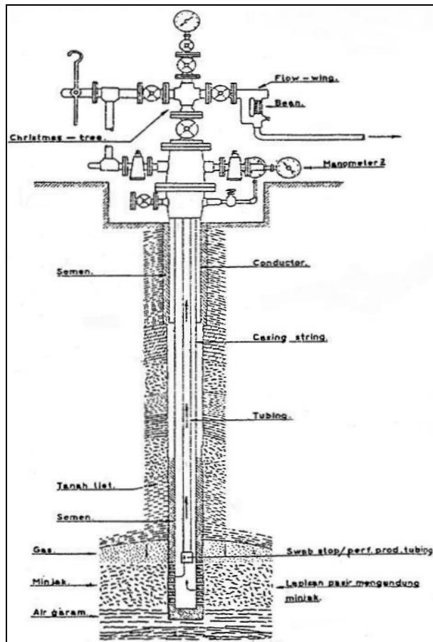
Gambar 8.5. Instalasi Sumur Sembur Alam
