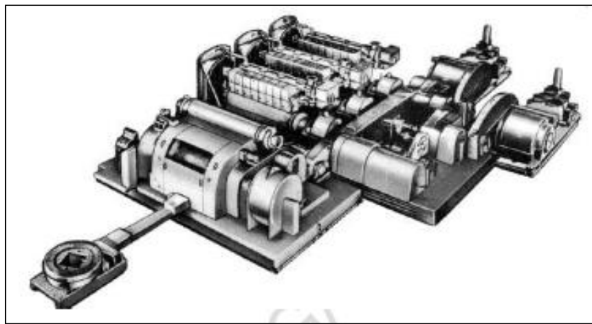
Gambar 4.13. Rotary table dengan penggerak Drawwork
