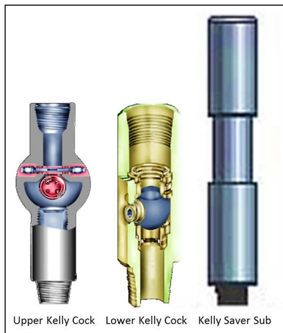
Gambar 4.25. Perlengkapan Kelly
