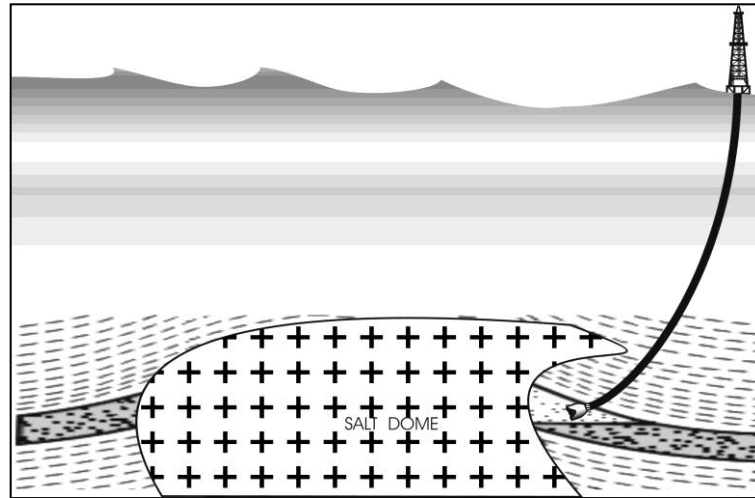
Gambar 3.9. Formasi dibawah Kubah Garam
