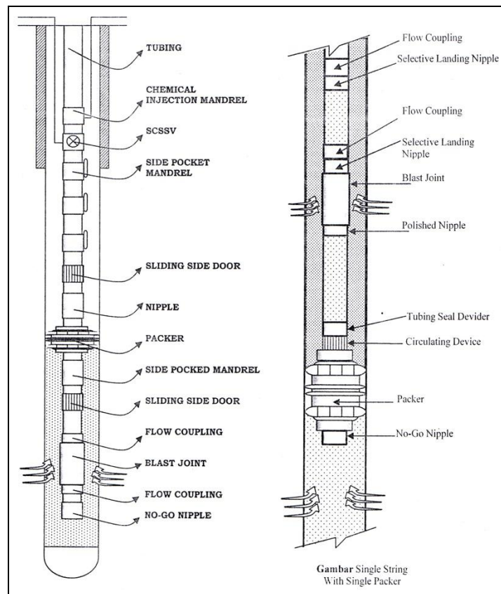
Gambar 8.6 Instalasi Bawah permukaan sumur sembur alam
