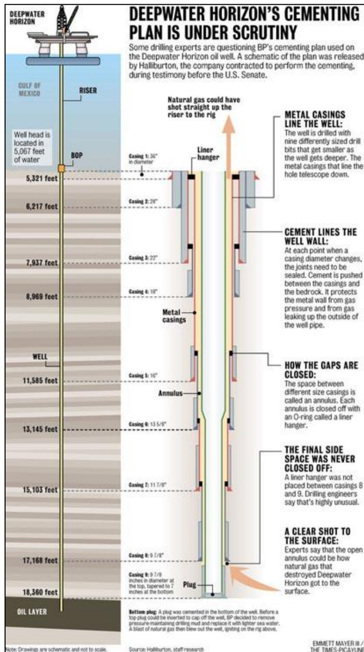
Gambar 5.1. Contoh Konstruksi Sumur Pengeboran
