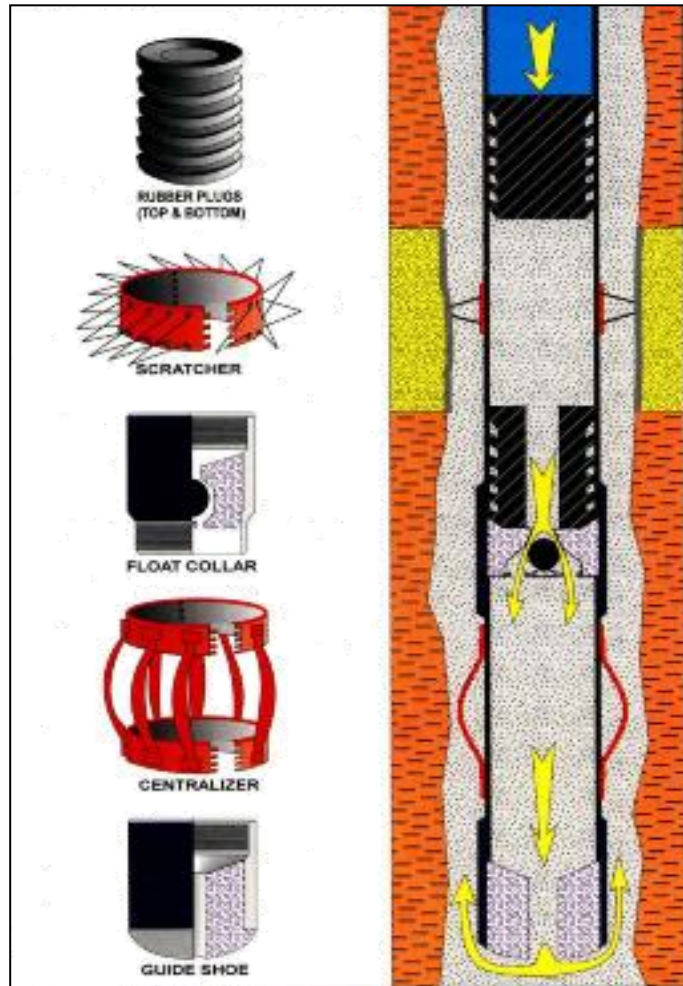
Gambar 5.10. Peralatan Bawah Permukaan
