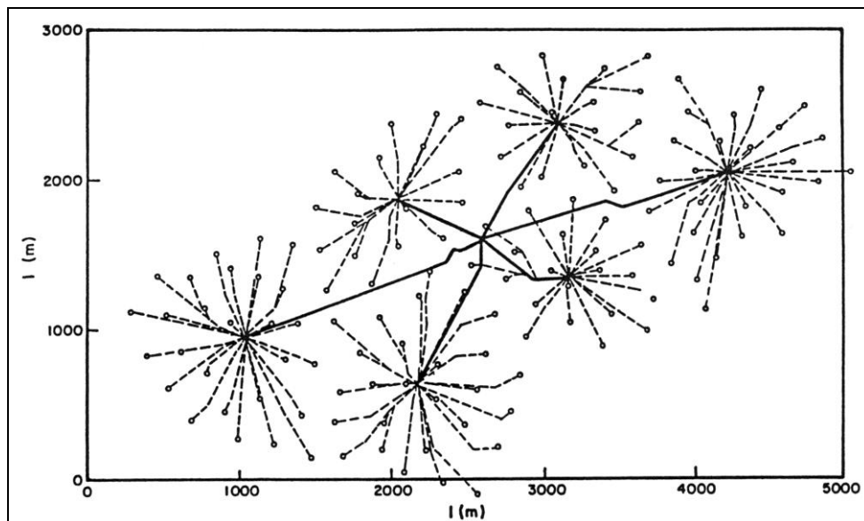
Gambar 8.13. Sistim Optimasi Gathering
