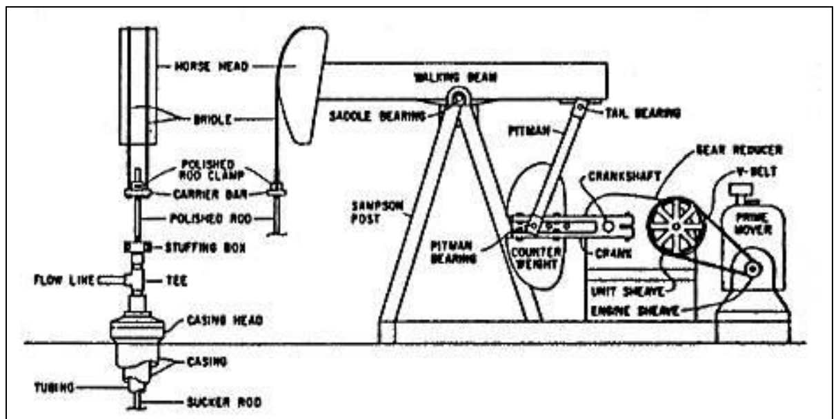
Gambar 8.9. Peralatan Permukaan Suatu Instalasi Pemompaan Beam
