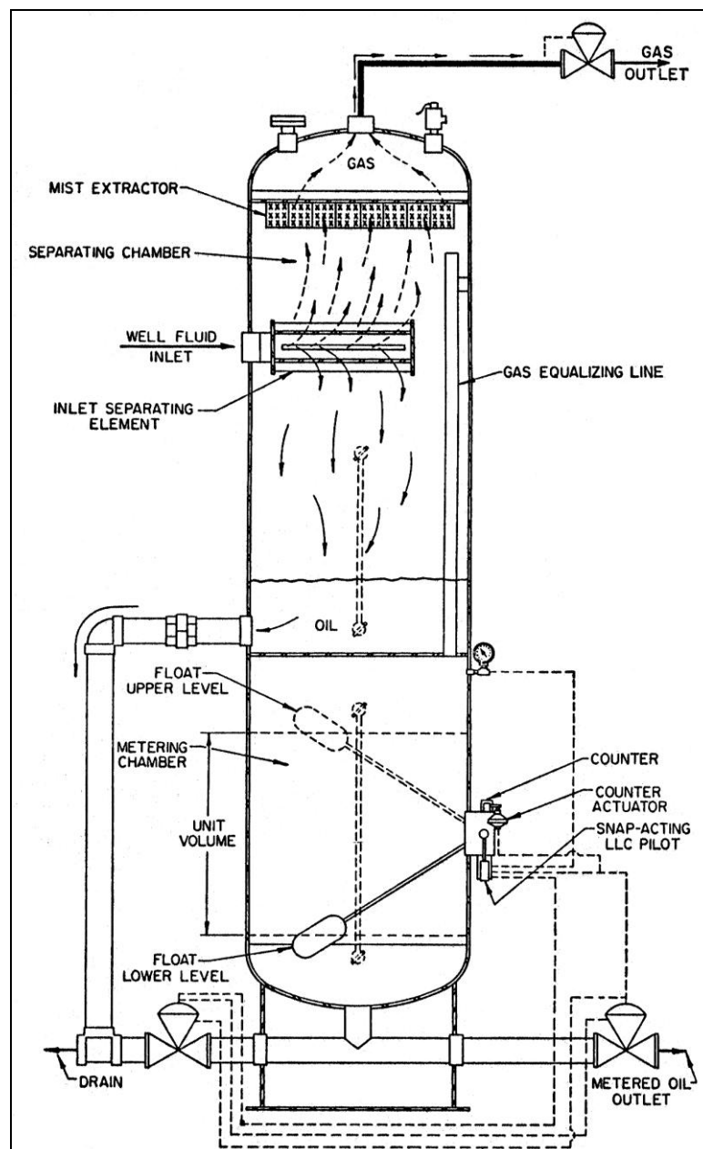
Gambar 8.15. Skema Separator Vertikal
