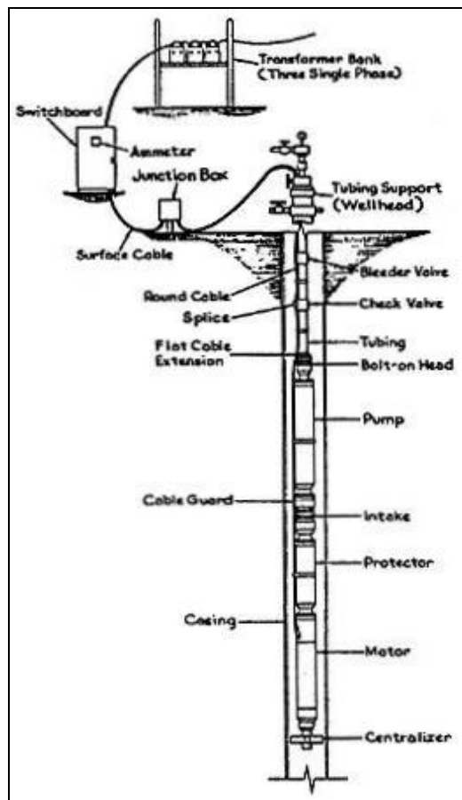
Gambar 8.10. Unit Pemompaan ESP
