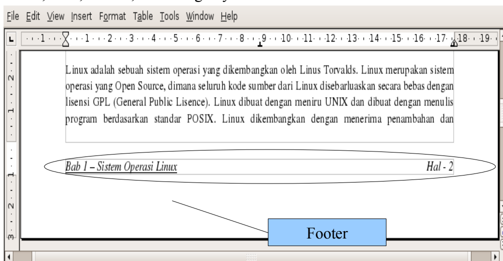
Gambar 3.4 Footer
