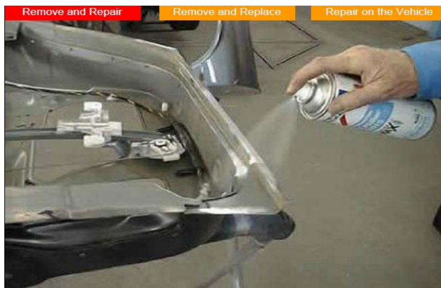
Gb.2.3. Pelapisan primer coating pada seluruh permukaan pelindung (guard)
