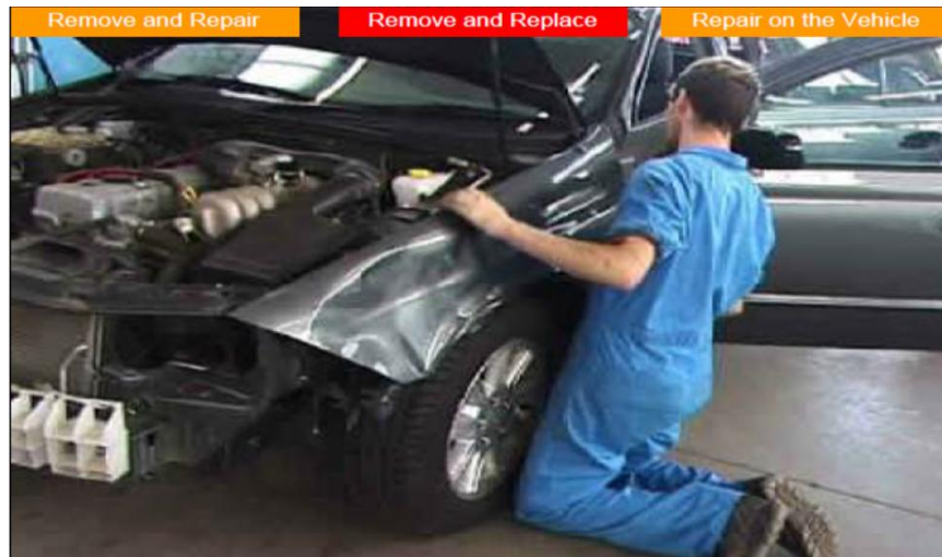
Gb.1.17. Pelepasan fender
