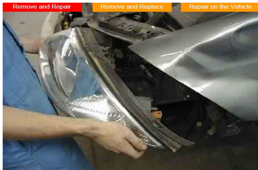
Gb.1.10. Pelepasan rangkaian lampu kepala
