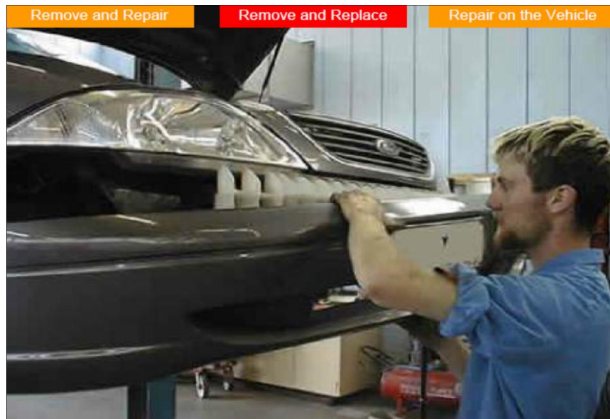
Gb.1.9. Pelepasan bumper
