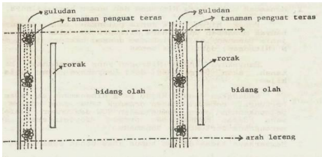
Gambar 51. Penampang membujur rorak
