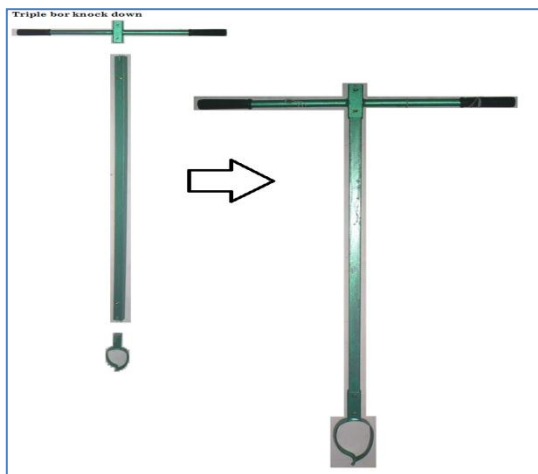
Gambar 45. Alat/bor biopori model biasa yang diproduksi awal
