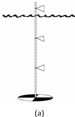
Gambar 28. Pengukuran kecerahan (a) secchi disk dengan skala pengukuran dan (b) penggunaan secchi disk
