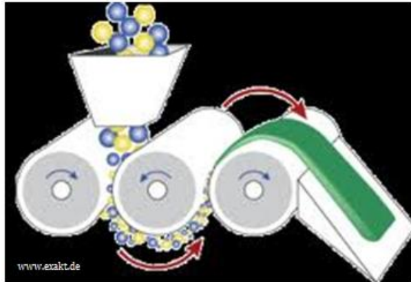
Gambar 16. Gambar prinsip kerja roll mill .
