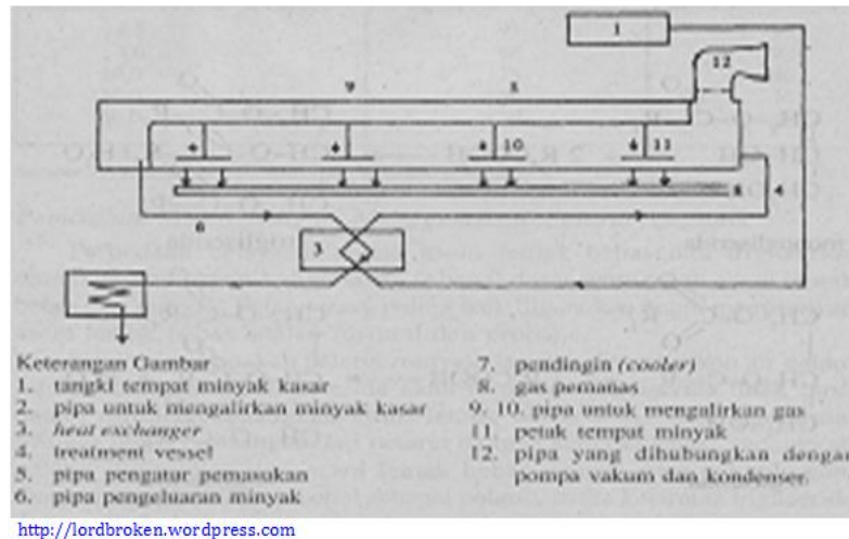
Gambar 64. Gambar skema alat penyulingan asam lemak bebas.
