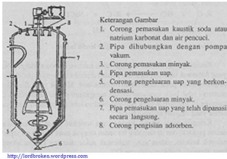
Gambar 63. Gambar alat netralisasi dan pemucatan minyak.
