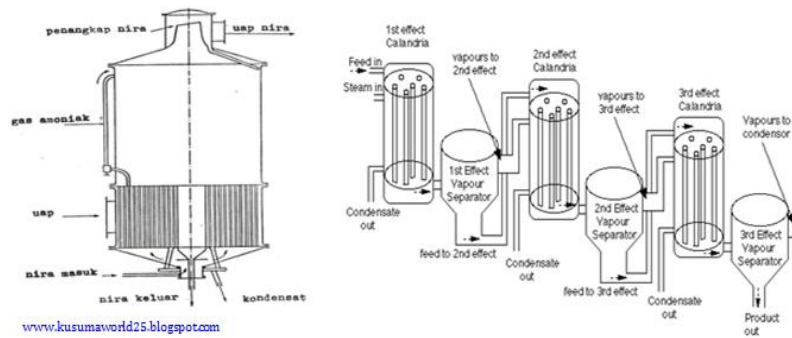
Gambar 43. Evaporator efek majemuk pada pembuatan nira.
