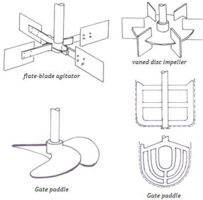
Gambar 23. Jenis-jenis alat pengaduk (agitator) (Lily, 2012)
