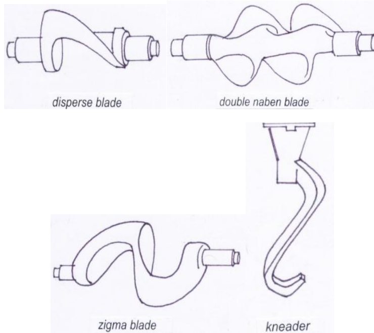
Gambar 28. Jenis-jenis pengaduk untuk pasta atau adonan (Lily, 2012)
