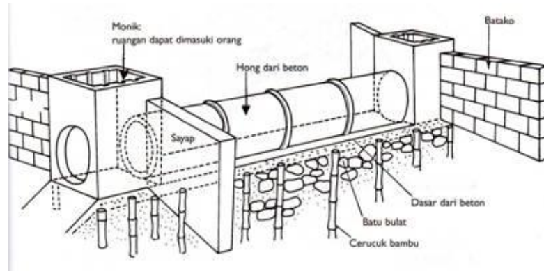
Gambar 48. Konstruksi pintu monik 1
