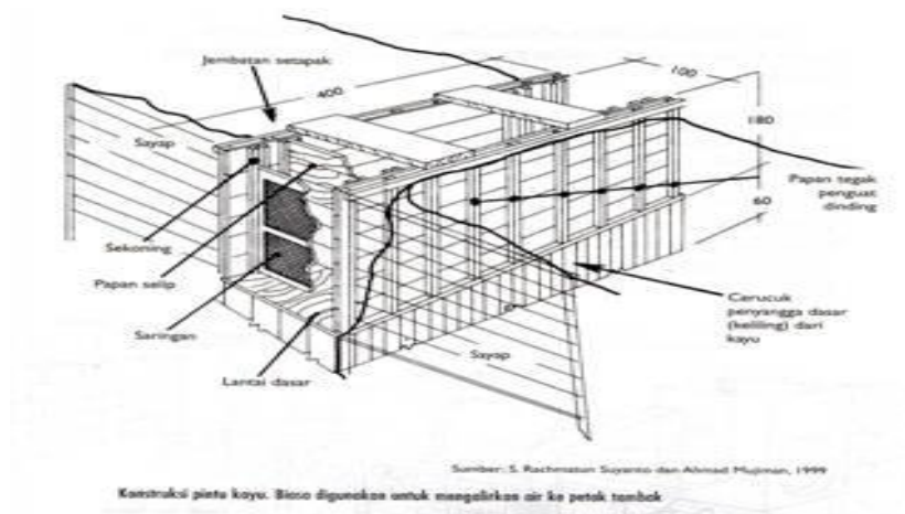
Gambar 49. Konstruksi pintu kayu 1
