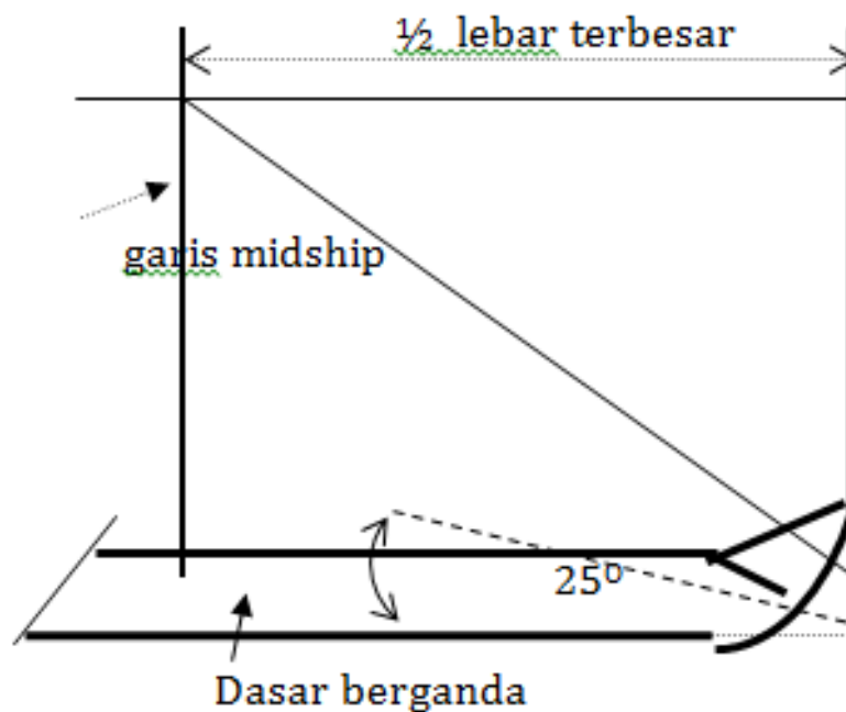
Gambar 14. Tinggi dasar berganda
