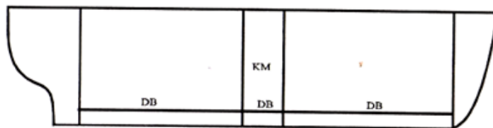
Gambar 13. Panjang Dasar Berganda kapal ≥ 76 m
