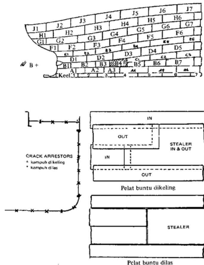
Gambar 16. Kulit Kapal
