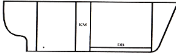
Gambar 11. 50 m < Panjang Dasar Berganda kapal < 61 m
