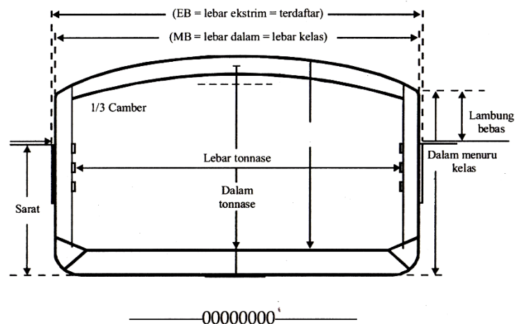
Gambar 3. ukuran melintang/melebar (transverzal) dan tegak (vertical)
