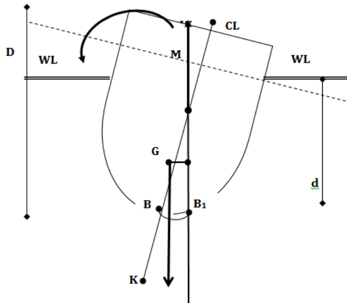
Gambar 19. Titik-titik penting dalam stabilitas
