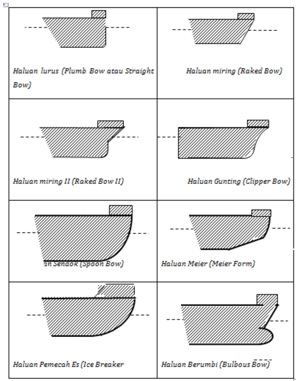
Gambar 6. Jenis-jenis Haluan Kapal
