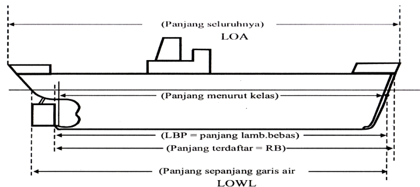
Gambar 2. Ukuran membujur/memanjang (longitudinal)
