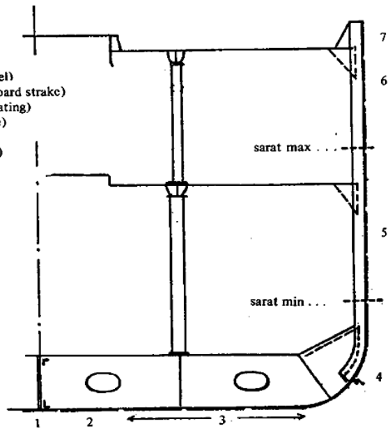
Gambar 15. Nama-nama kulit kapal
