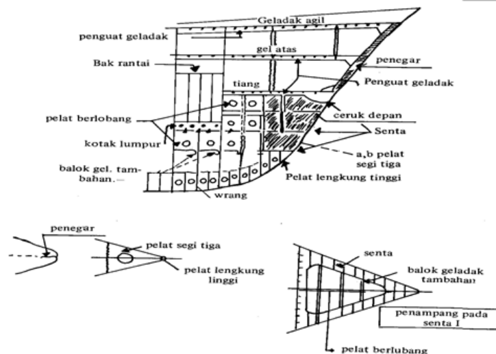
Gambar 4. Penampang membujur haluan
