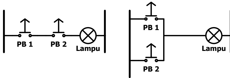
Gambar7 Rangkaian AND dan OR.
