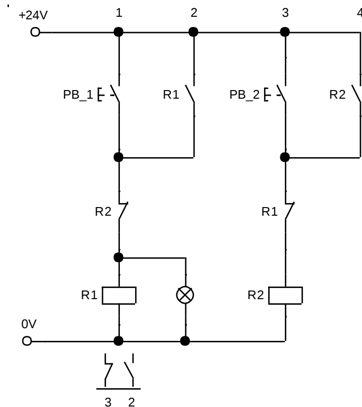
Gambar 10 Rangkaian interlock
