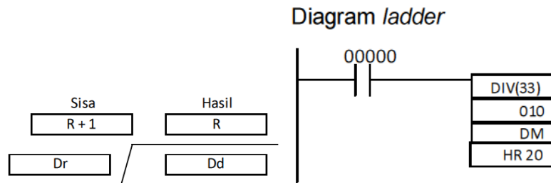
Gambar 47 Program aritmatik pembagian.
