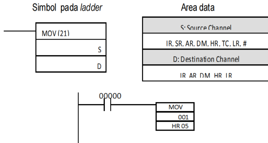
Gambar 48 Simbol dan Area data MOV dan diagram Ladder MOV.
