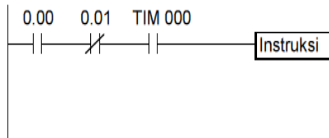
Gambar 22 Instruksi AND dan AND NOT
