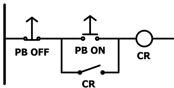
Gambar 8 Rangkaian pengunci.
