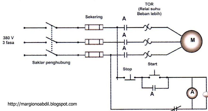
Gambar 5 Diagram kelistrikan secara horizontal
