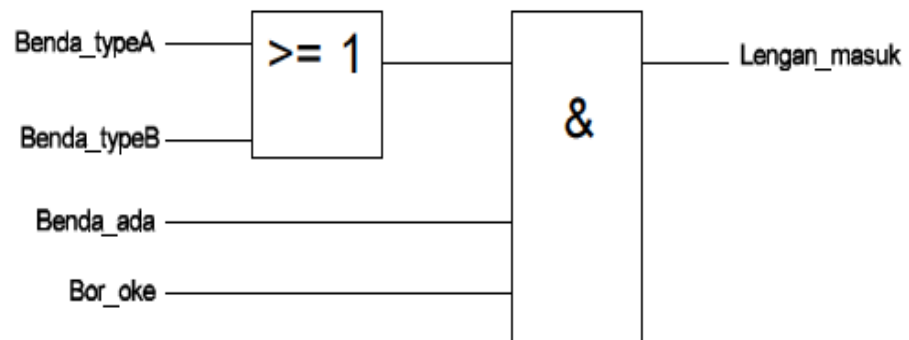
Gambar 17 Pemrograman dengan Function Blok Diagram.
