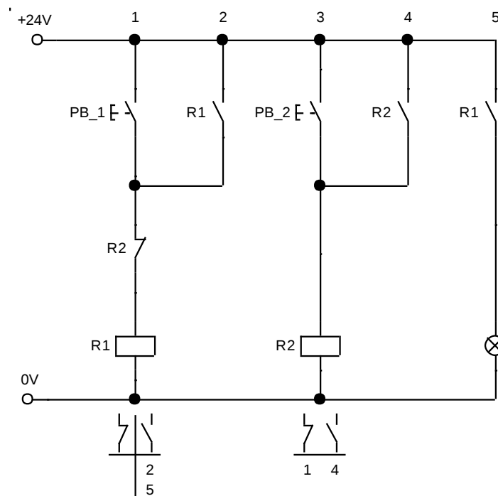
Gambar 9 Rangkaian pengaman
