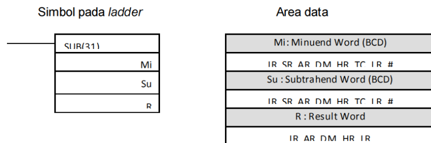
Gambar 42 Simbol dan Area data SUB.
