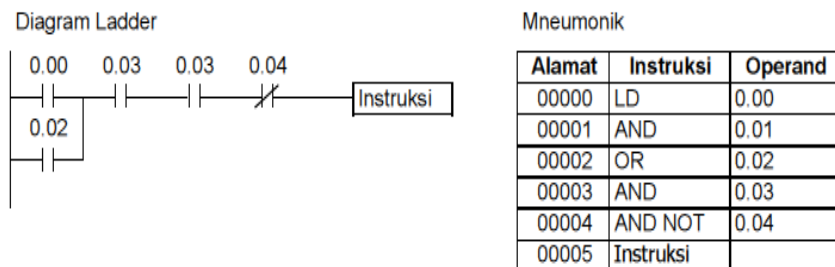
Gambar 24 Instruksi AND dan OR
