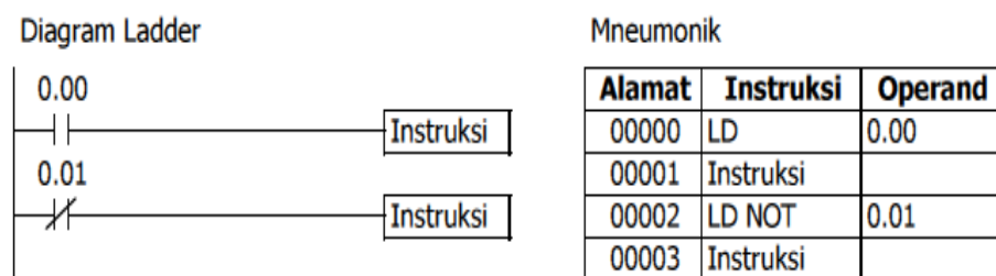
Gambar 18 Pemrograman dengan Statement List.
