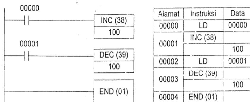
Gambar 39 Program INC dan DEC
