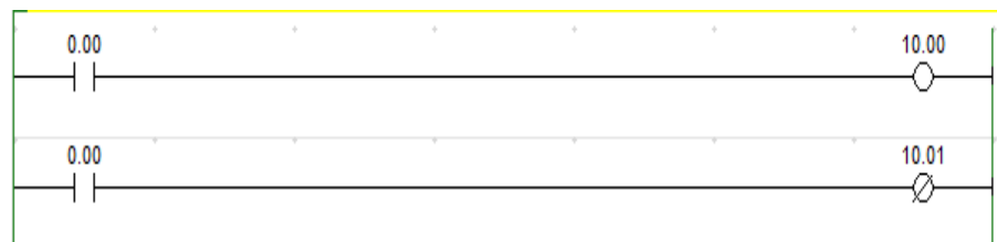
Gambar 25 Instruksi OUT dan OUT NOT
