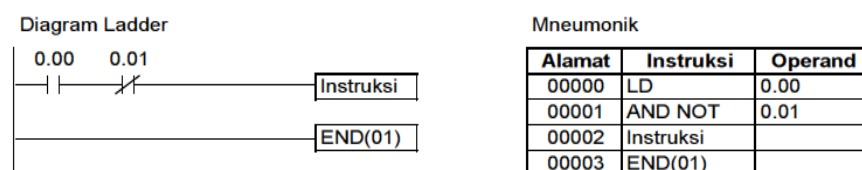
Gambar 26 Instruksi END (01)
