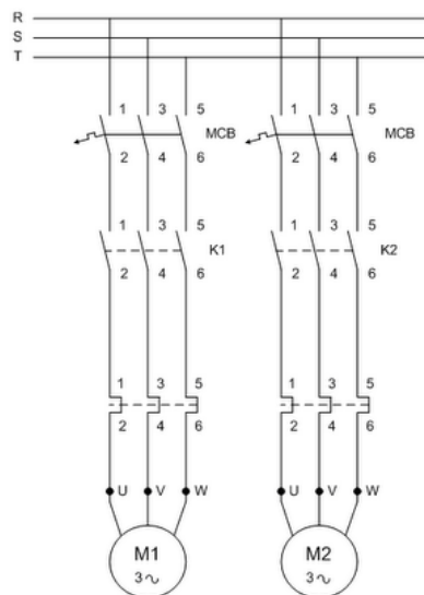
Gambar 88 Diagram Daya 2 Motor 3 Phasa Menyala Berurutan
