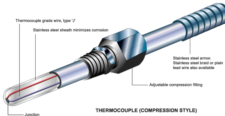
Gambar 30. Termokopel
