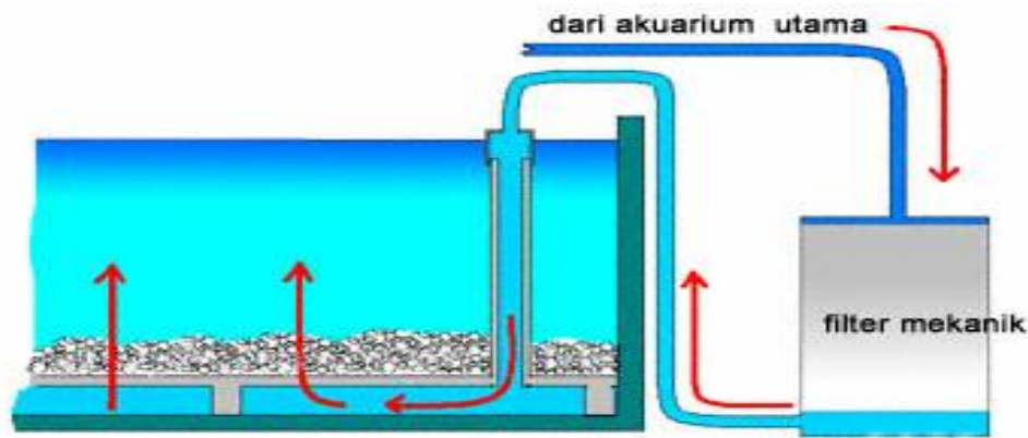
Gambar 7. Filter under gravel dengan aliran air terbalik.
