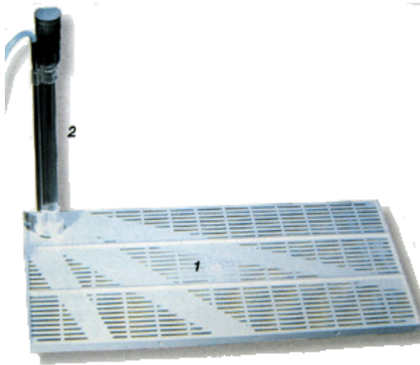
Gambar 5. Contoh Konstruksi Filter "Under Gravel".
