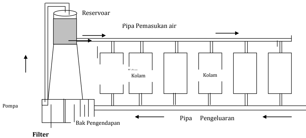
Gambar 103 Skema Pembesaran Ikan pada sistem Resirkulasi
