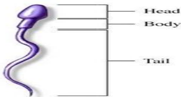
Gambar 94. Sperma Ikan
