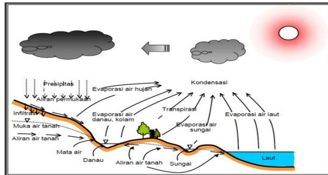
Gambar 8. siklus air
