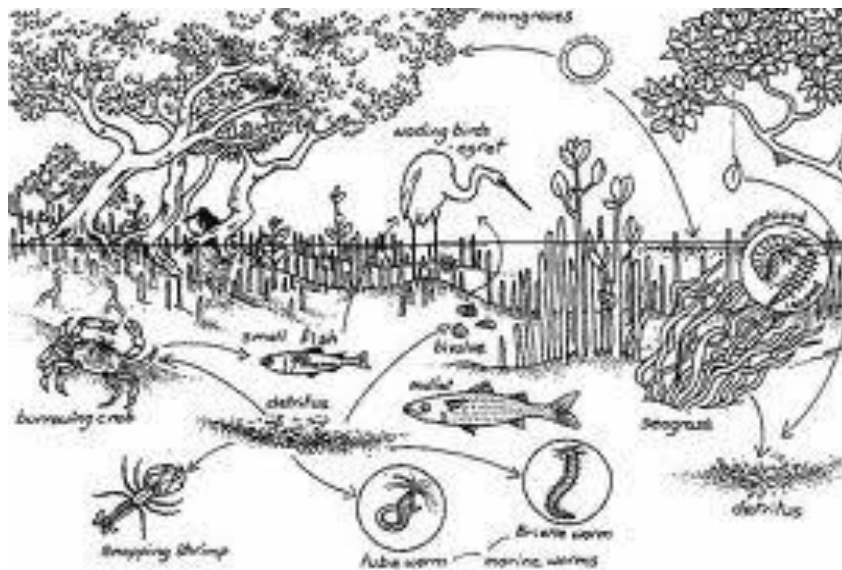
Gambar 2. Perpindahan energi
