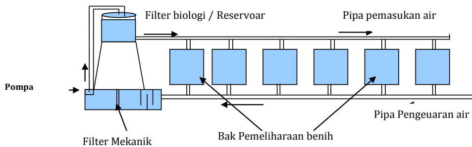
Gambar 88. Resirkulasi Air
