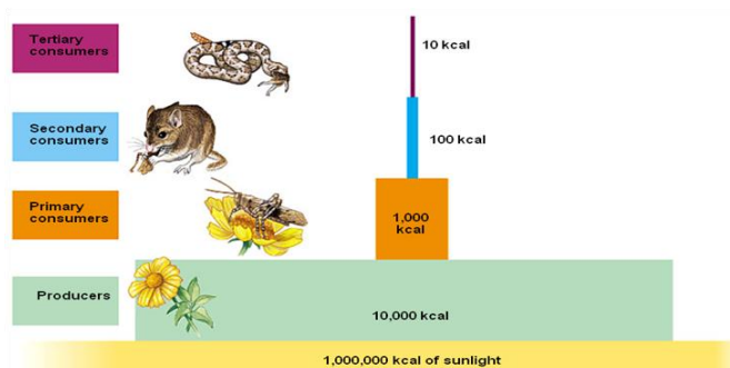
Gambar 33. Aliran Energi
