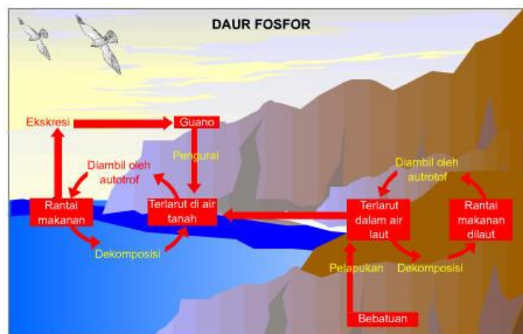
Gambar 49. Siklus Fosfor
