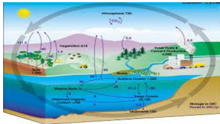
Gambar 50. Siklus Karbondioksida
