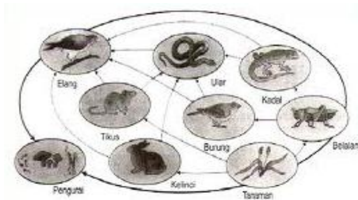
Gambar 44. Jaring Makanan
