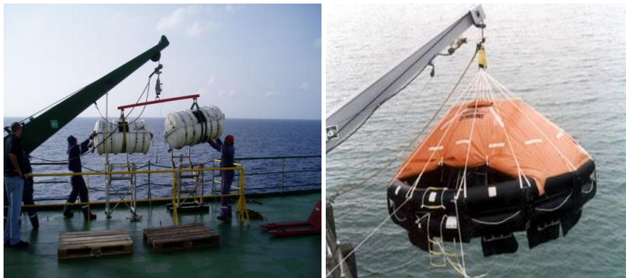
Gambar 68. Jenis rakit penolong yang diturunkan menggunakan davit
