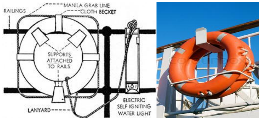
Gambar 38. Penyimpanan lifebuoy pada tempatnya agar dapat terlepas sendiri
