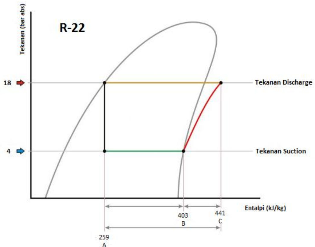
Gambar 1.3 Pemetaan Siklus Refrijerasi Unit Tata Udara
