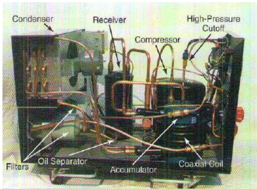
Gambar 5.8 Konstruksi Mesin recovery
