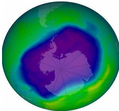
Gambar 5.2. Lubang Ozon semakin Membesar di Antartika
