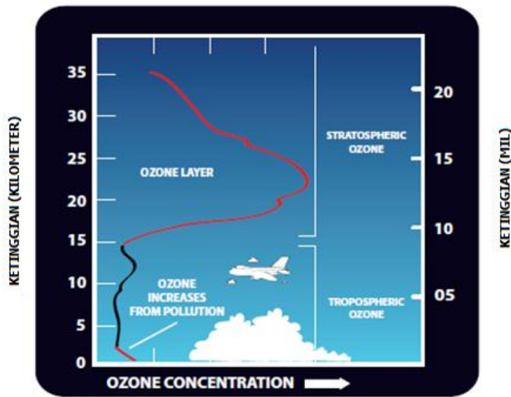
Gambar 5.1 Distribusi Ozon di Atmosfir
