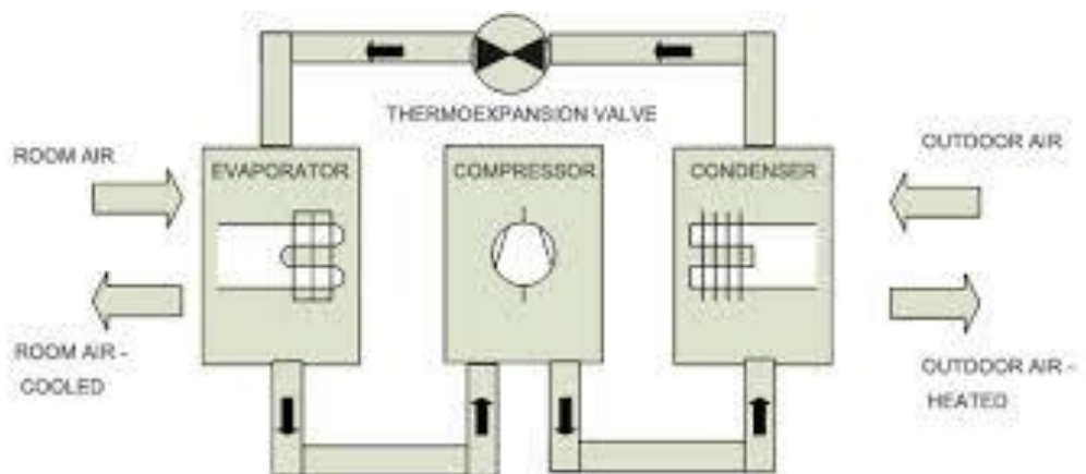
Gambar 3.1 Proses Penukaran Kalor pada Unit Tata Udara
