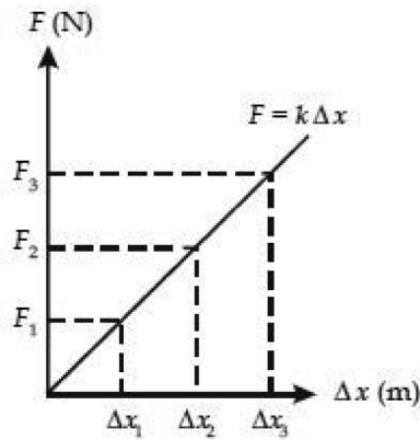
Gambar 6.3 Grafik hubungan terhadap Δx pada kurva F = k\Delta x .
