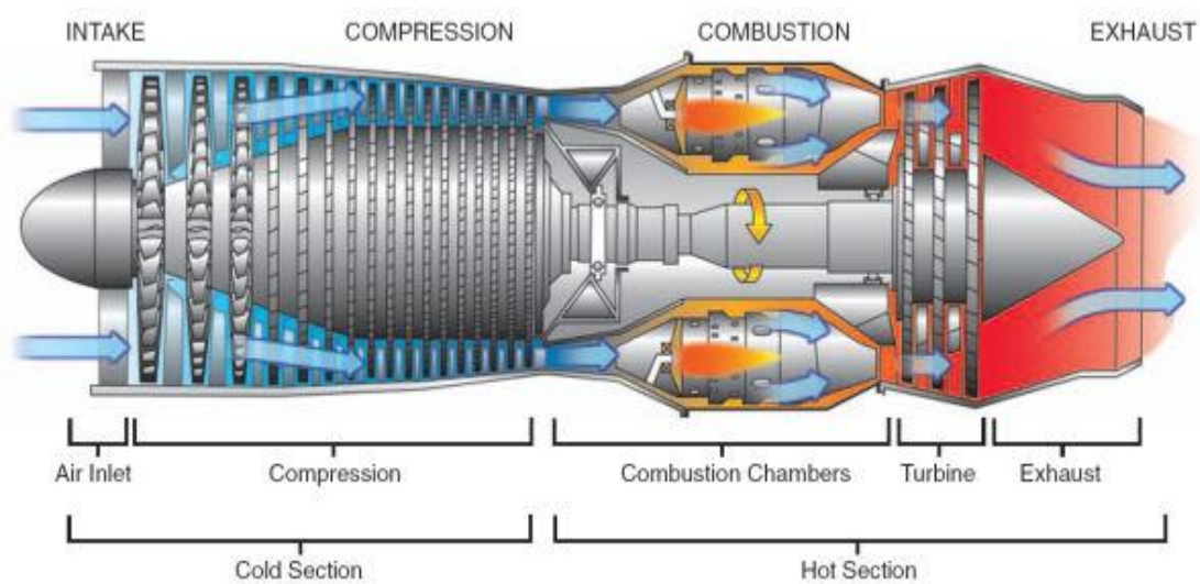
Gambar -3 Bagian utama motor Turbojet
