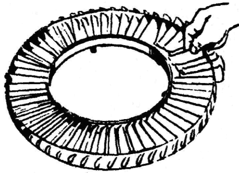
Gambar 50. Rakitan nosel turbin dengan sudu sudu yang dapat dilepas
