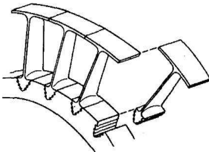
Gambat 53. Bucket turbin metoda pengikatan tang pemasangan sudu sudu turbin.
