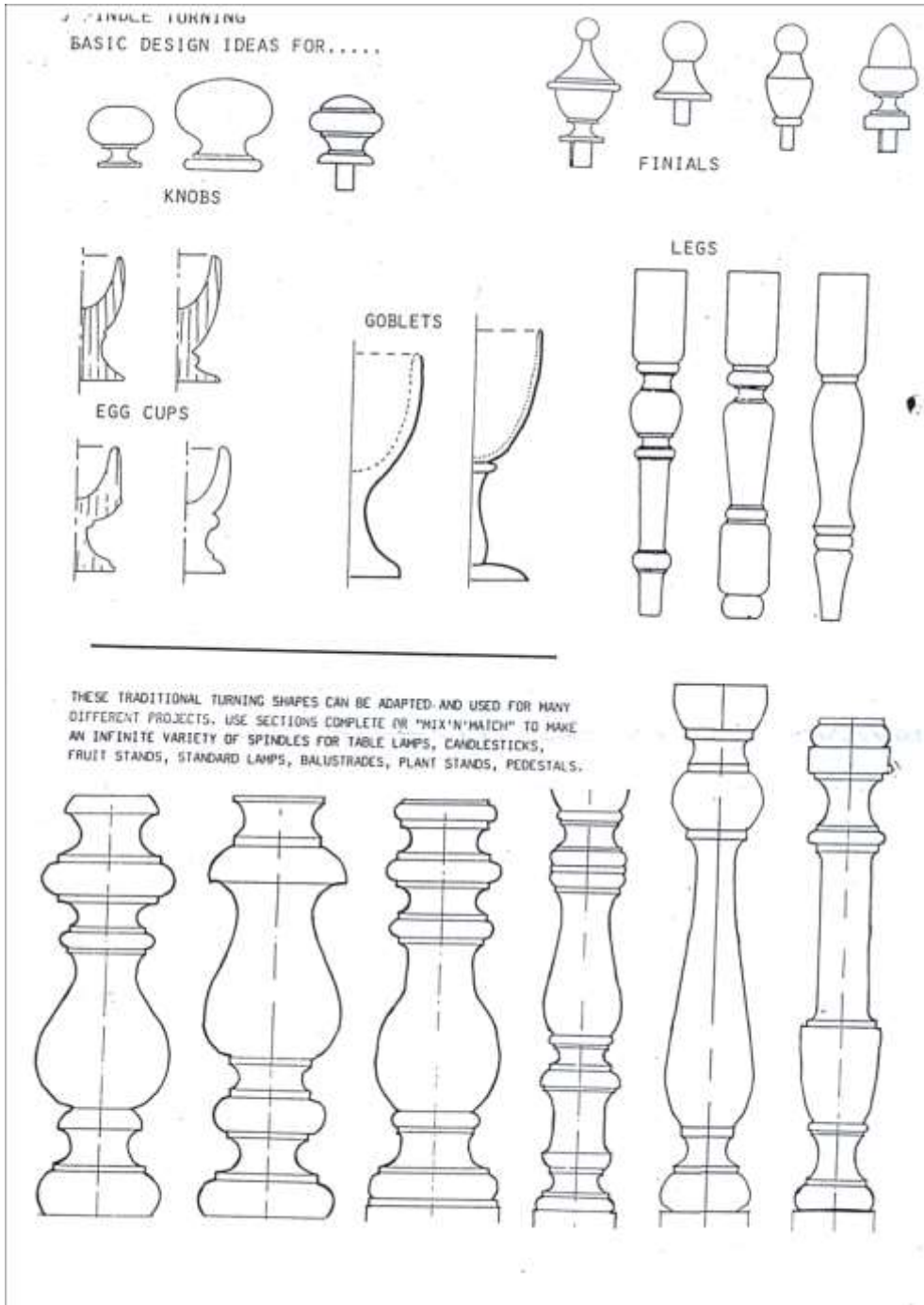
(Gambar 4-19. Gambar kerja teknik cembung, cekung dan alur) Sumber Dok. Studio Kayu
