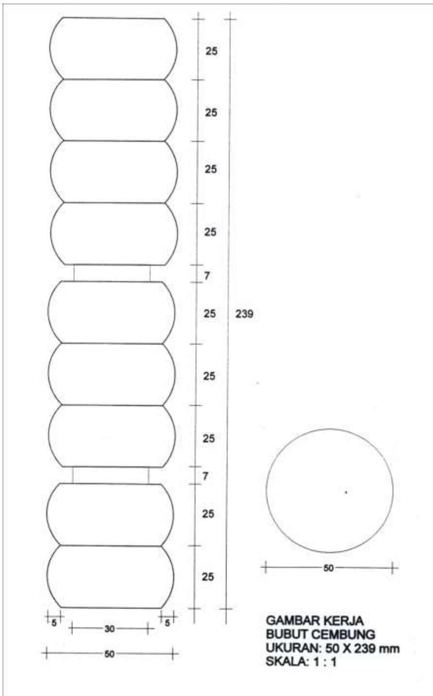
(Gambar 4.15. Gambar kerja profil cembung) Sumber dok. Studio Kayu
