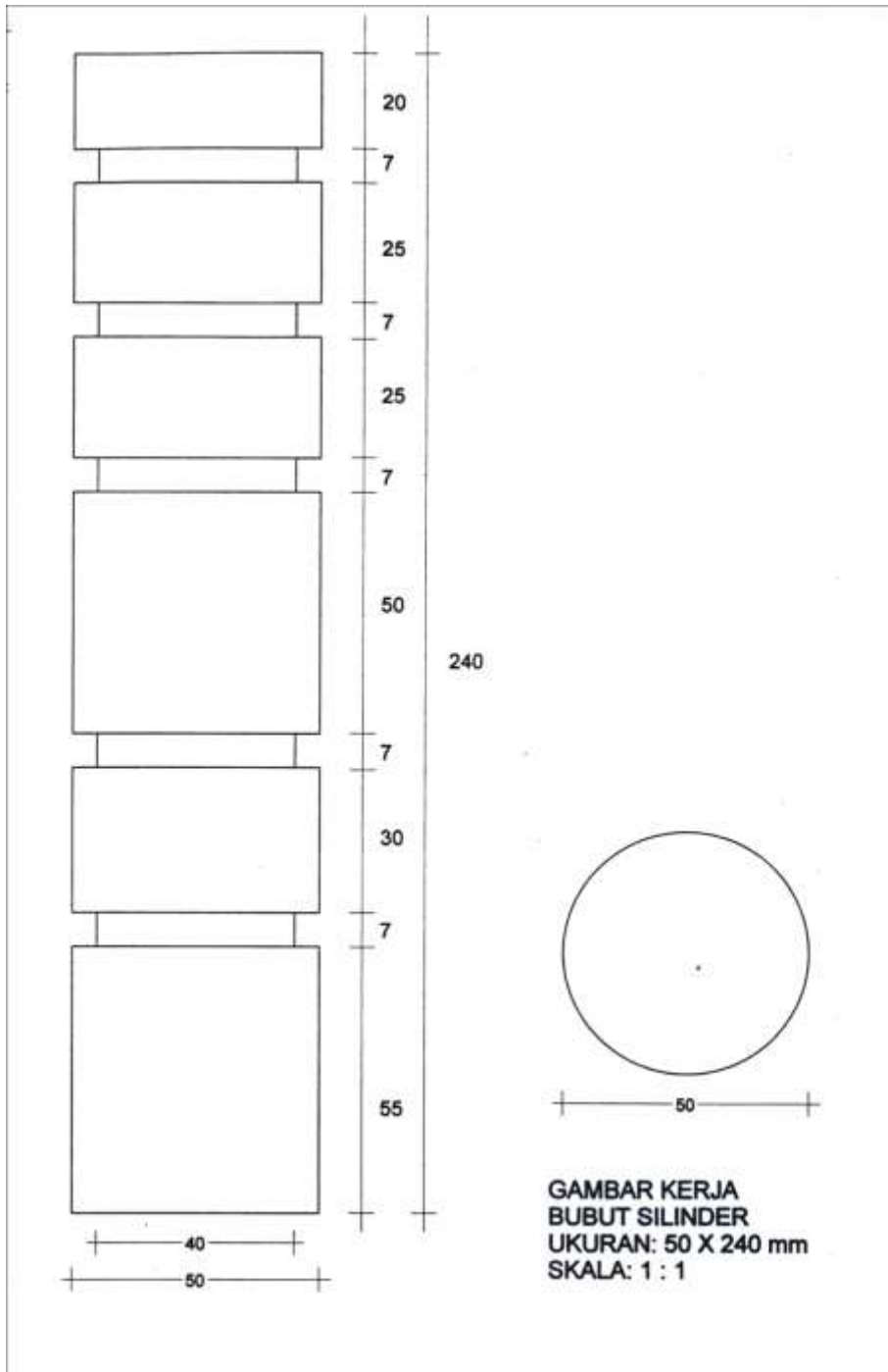
(Gambar 4.16. Gambar kerja profil alur) Sumber dok. Studio Kayu
