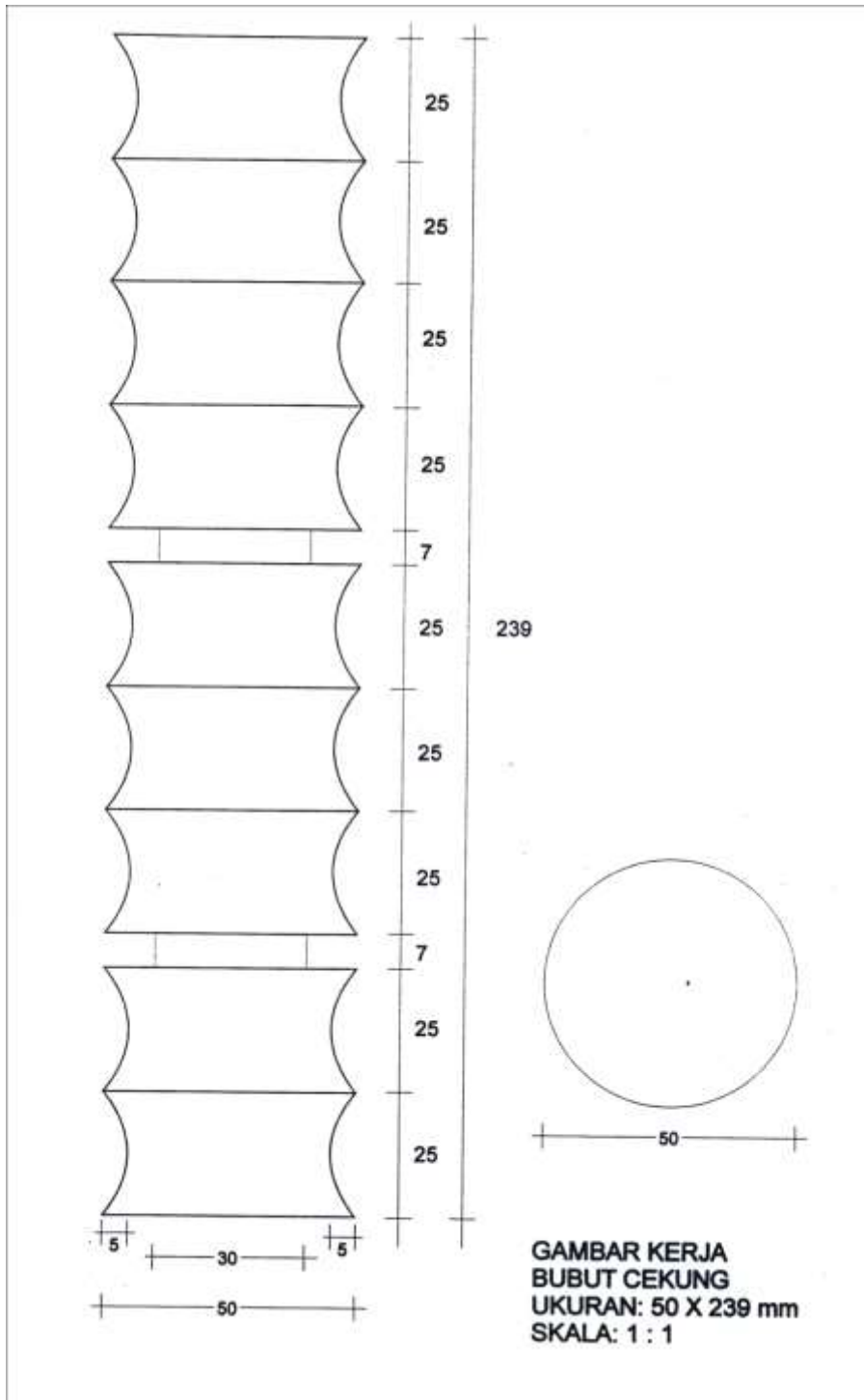
(Gambar 4.14. Gambar kerja profil cekung) Sumber dok. Studio Kayu
