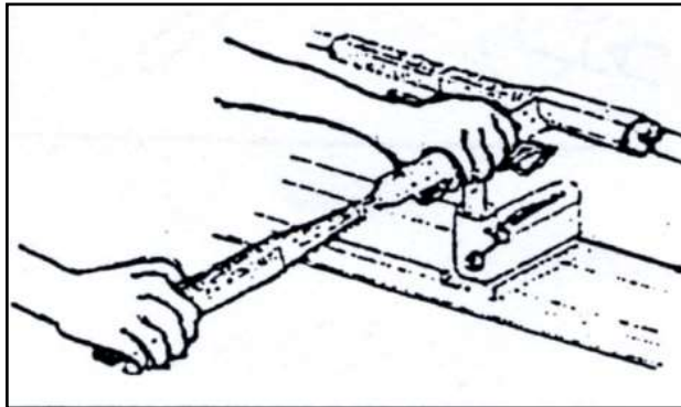
(Gambar 4-4. Pembentukan awal) Sumber dok. Studio Kayu
